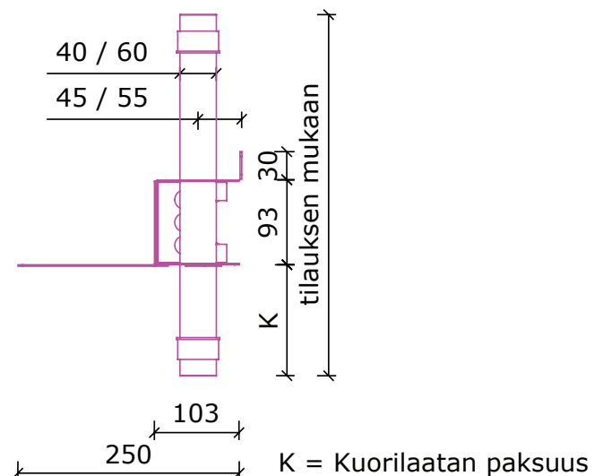
SIVUKUVA
