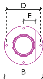
PÄÄTYKAPPALE PÄÄLTÄ
